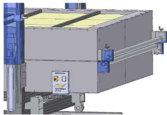
Dettaglio della zona dei rulli di uscita a forno chiuso
